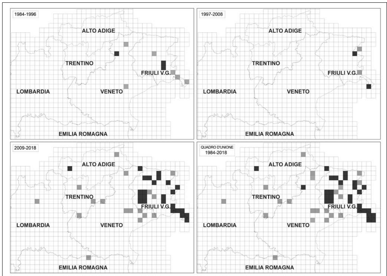
Fig. 1. Attuale distribuzione di Canis aureus in Italia in base ai soli dati di C1 (sensu HATLAUF et al. , 2016). Reticolo cartografico ETRS 1989 LAAEA con celle di 10x10 km.
